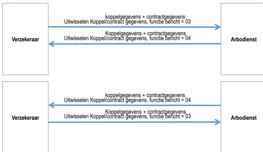
Figuur-6 Voorbeeld-2 uitwisselen koppel/contractgegevens
